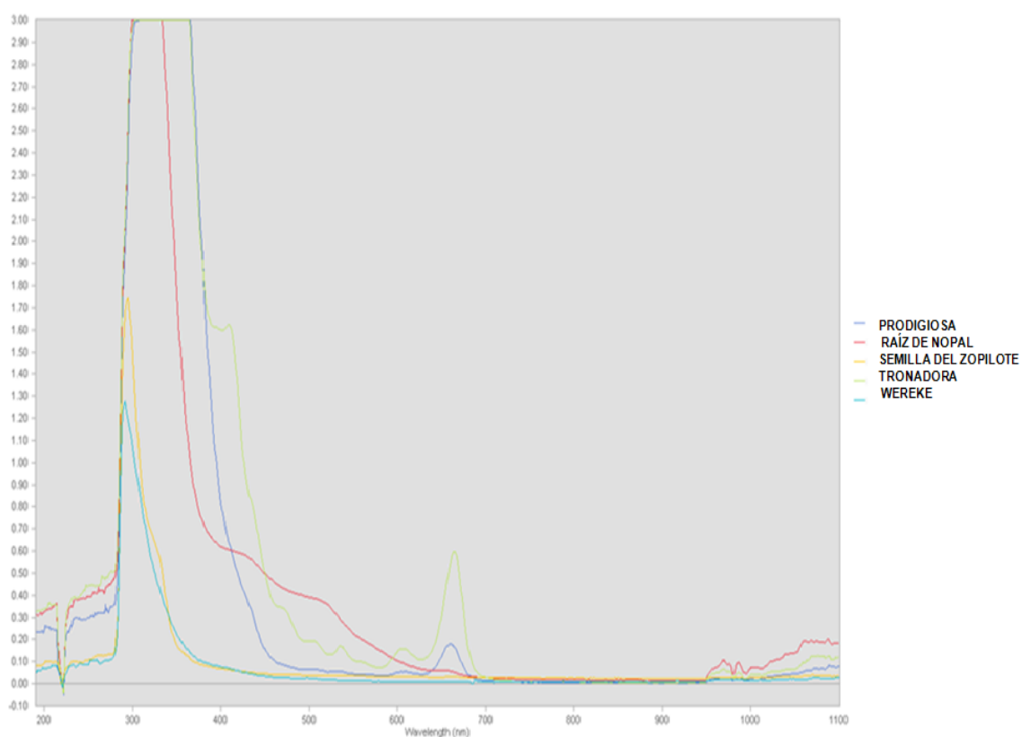
Figura 9. Huellas químicas empleando UV-Vis de los extractos metanólicos. En esta grafica se observa el patrón de absorción de los extractos de las plantas estudiadas.
